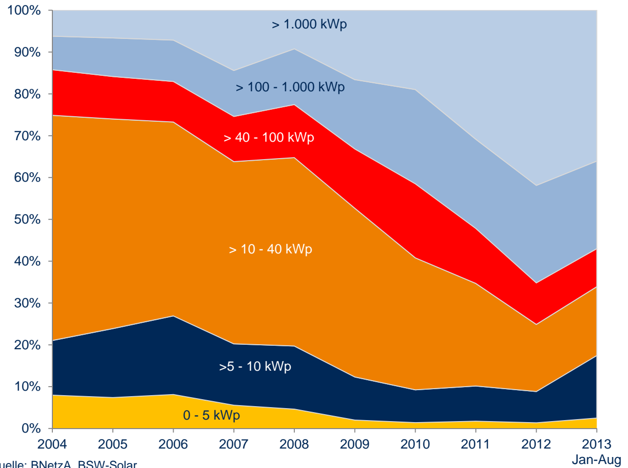
Photovoltaik-Zubau nach Anlagenklassen 2004 bis 2013 (bis August) Anteil kleiner PV-Anlagen nimmt bei schrumpfendem Markt zu, nach installierter Leistung
