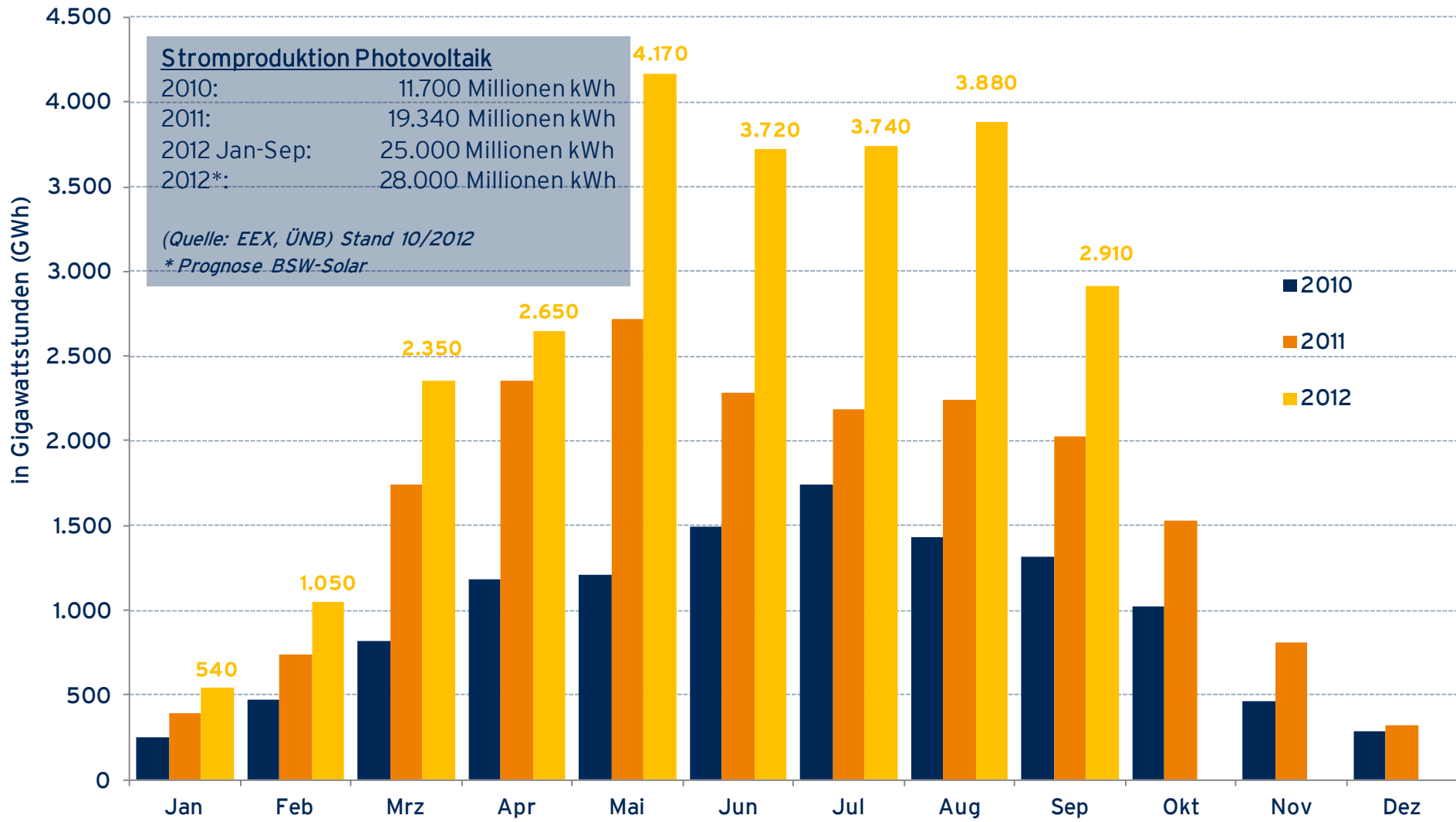
Quelle: ÜNB, EEX, eigene Berechnungen BSW-Solar 2012, vorläufige Hochrechnung, Stand 10/2012
