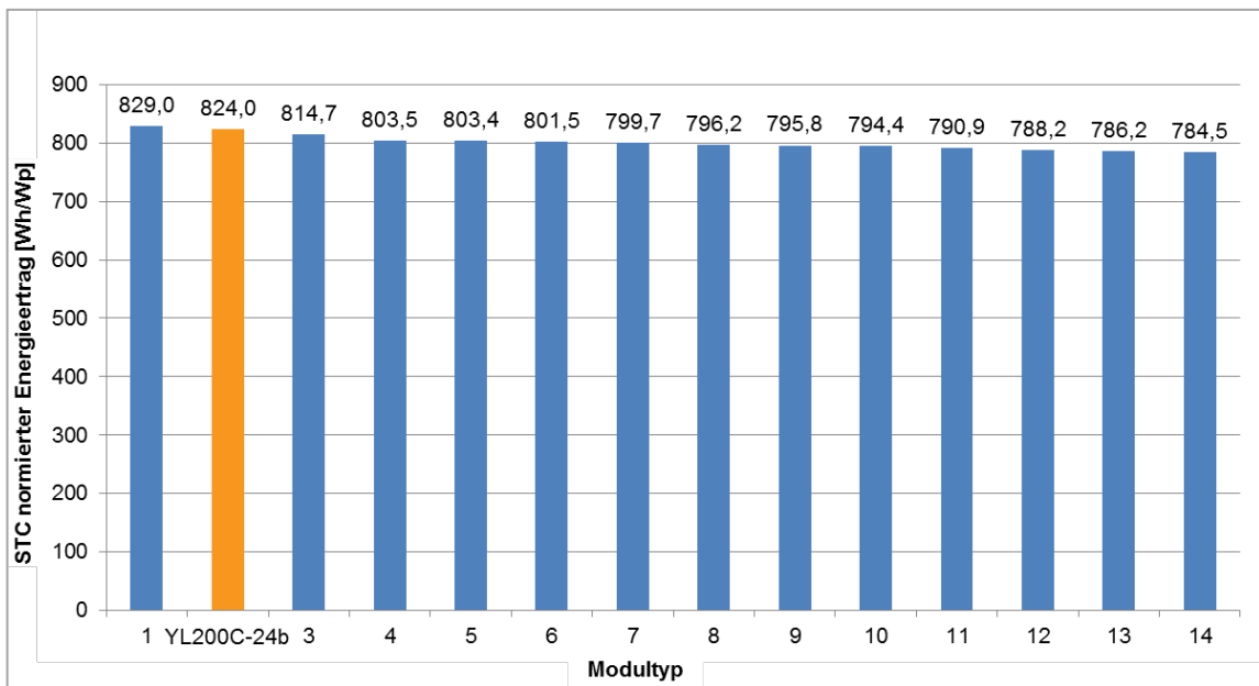
Abb. 1: Energieertrag, normiert auf die jeweilige Modulleistung unter Standardtestbedingungen (STC), von TÜV Rheinland gemessen (Zeitraum: 01.09.11 - 31.08.12).
